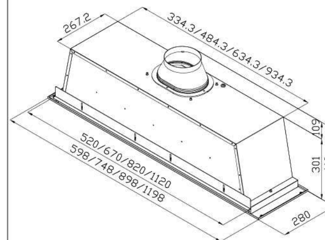
PQ-M60/75/90/120 BST 隱藏式
