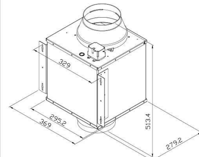
PB-850B 外掛式中繼馬達
