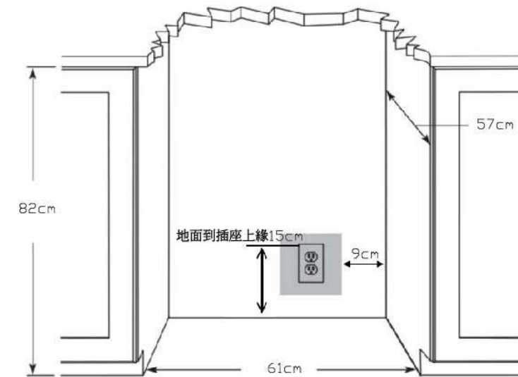
櫥下式紅酒櫃 預留空間尺寸圖
