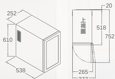
機體尺寸
