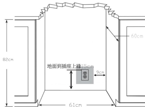
櫥下式紅酒櫃 預留空間尺寸圖
