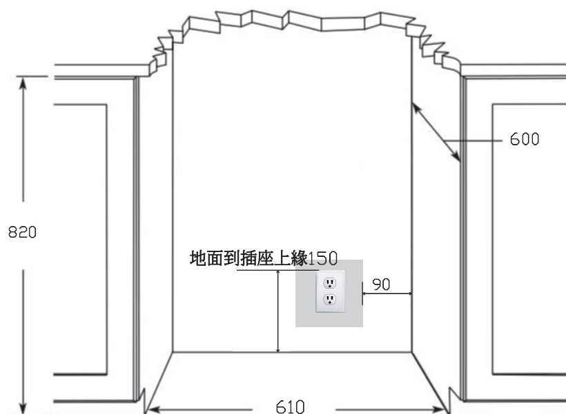
櫥下式紅酒櫃 預留空間尺寸圖
