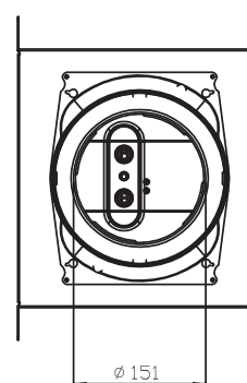
底端 (入風口)
