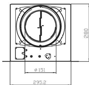
頂端 (出風口)
